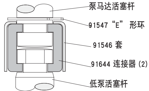
泵连接详图
