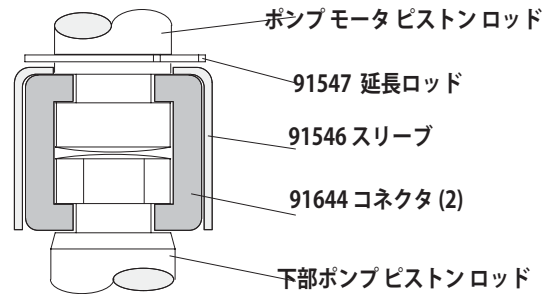
ポンプ接続詳細
